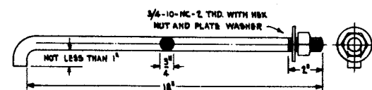
1157 - HOOK BOLT A.H.S.
