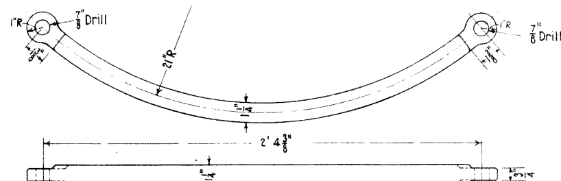
2682—90° DEFLECTING STAND BAR (O.H. STEEL)
